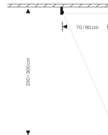
Empfohlener Wandabstand für homogene Wandaufhellung
